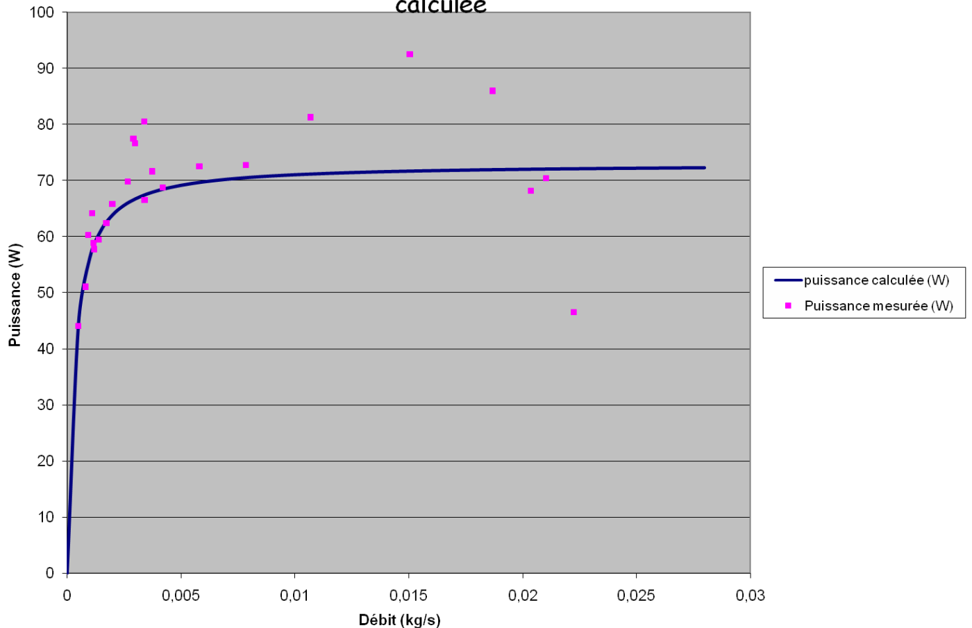
Comparaison de la Puissance thermique reçue par l'eau mesurée et calculée
