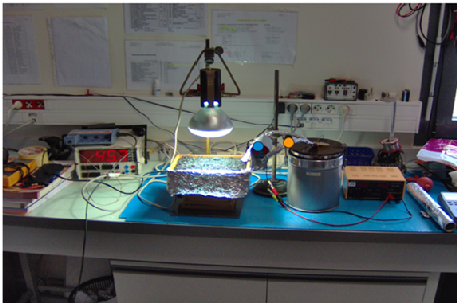
Troisième montage en circuit fermé
